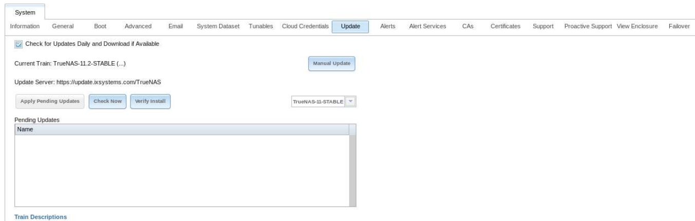
Fig. 4.12: Update Options
